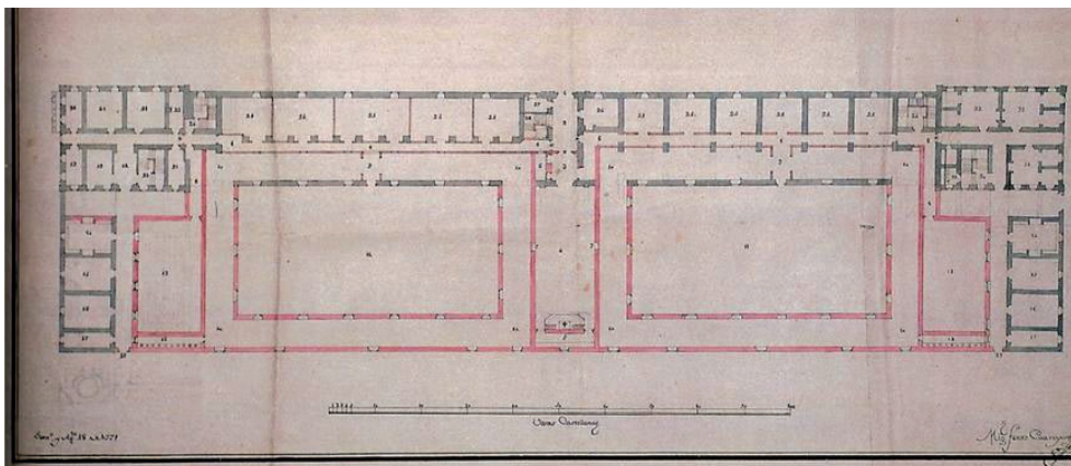
Figura 4 Hospicio de Pobres de Santiago de Compostela proyectado sobre el edificio antiguo cuartel de Santa Isabel (planta del piso bajo), Miguel Ferro Caaveyro, 1771. A.C.S.
